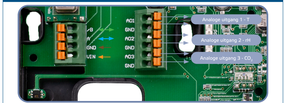
Fig. 4 Bedrading
