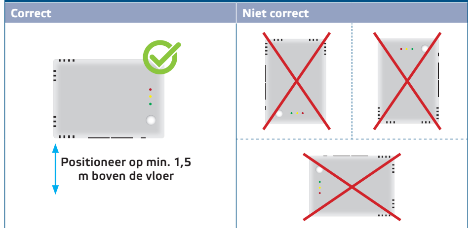
Fig. 3 Montagepositie
