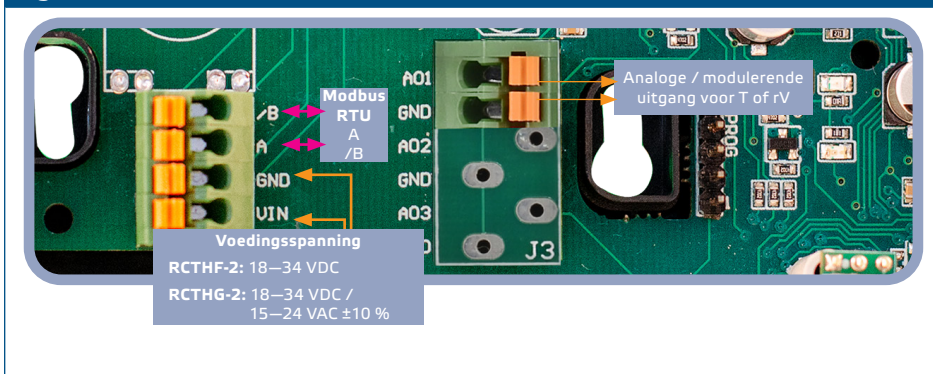
Fig. 4 Aansluitschema
