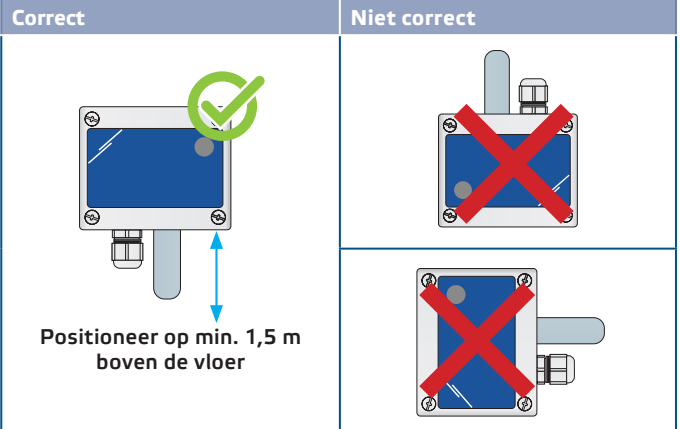
Fig. 2 Montagepositie
