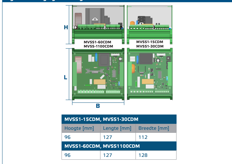
Fig. 1 Bevestiging Afmetingen
