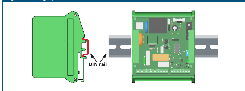
Fig. 2 Montage positie
