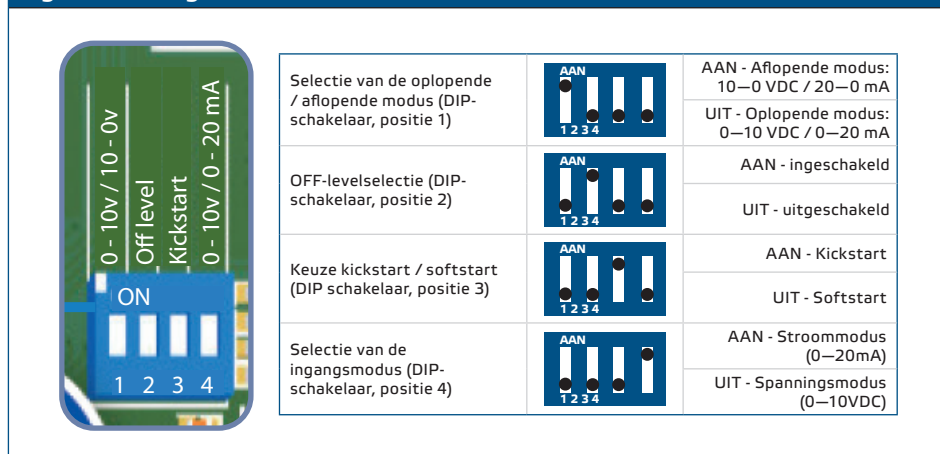
Fig. 4 Instellingen DIP-schakelaar
