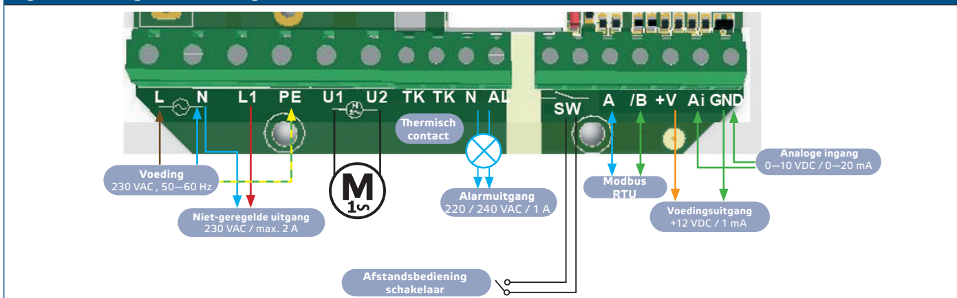
Fig. 3 Bedrading en aansluitingen
