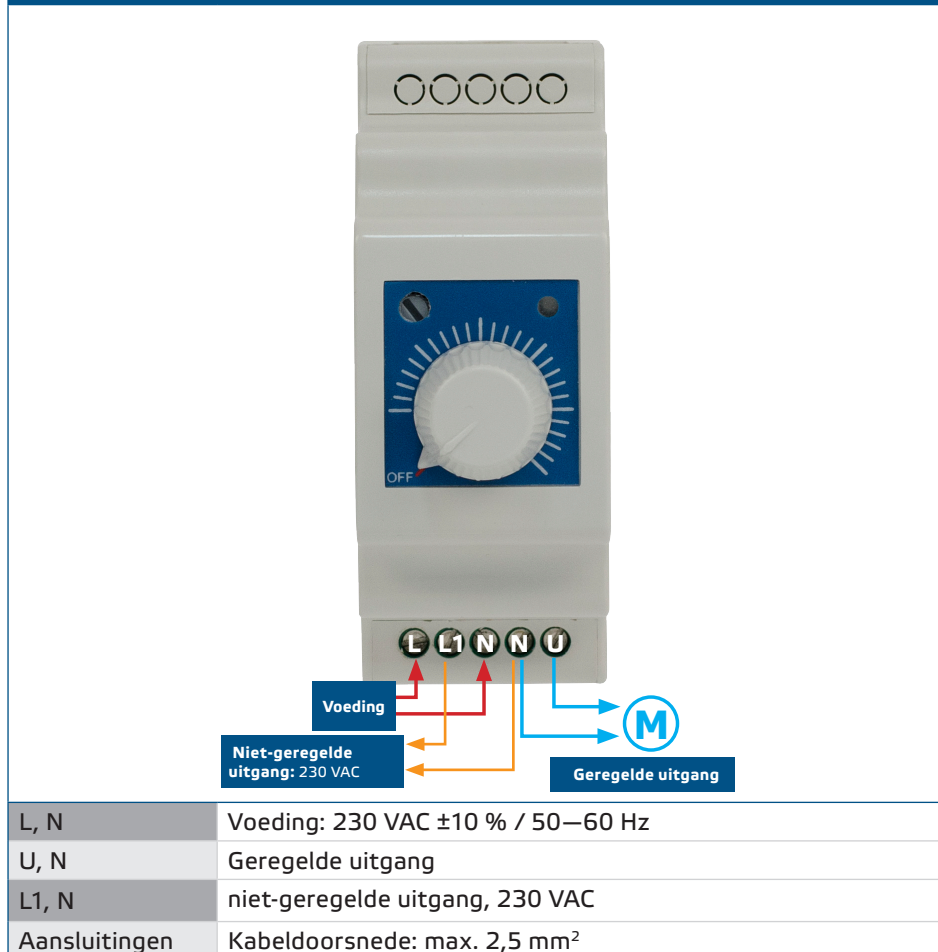
Fig. 1 Bedrading
