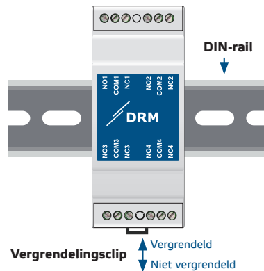
Fig. 2 Montagepositie
