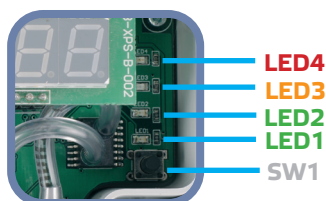
Fig. 7 Microschakelaar voor reset van de modbusregisters en voor de calibratie van de sensor
