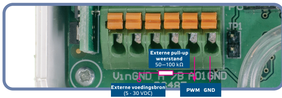
Fig. 6 PWM (Open collector) aansluiting (JP1 niet geplaatst)
