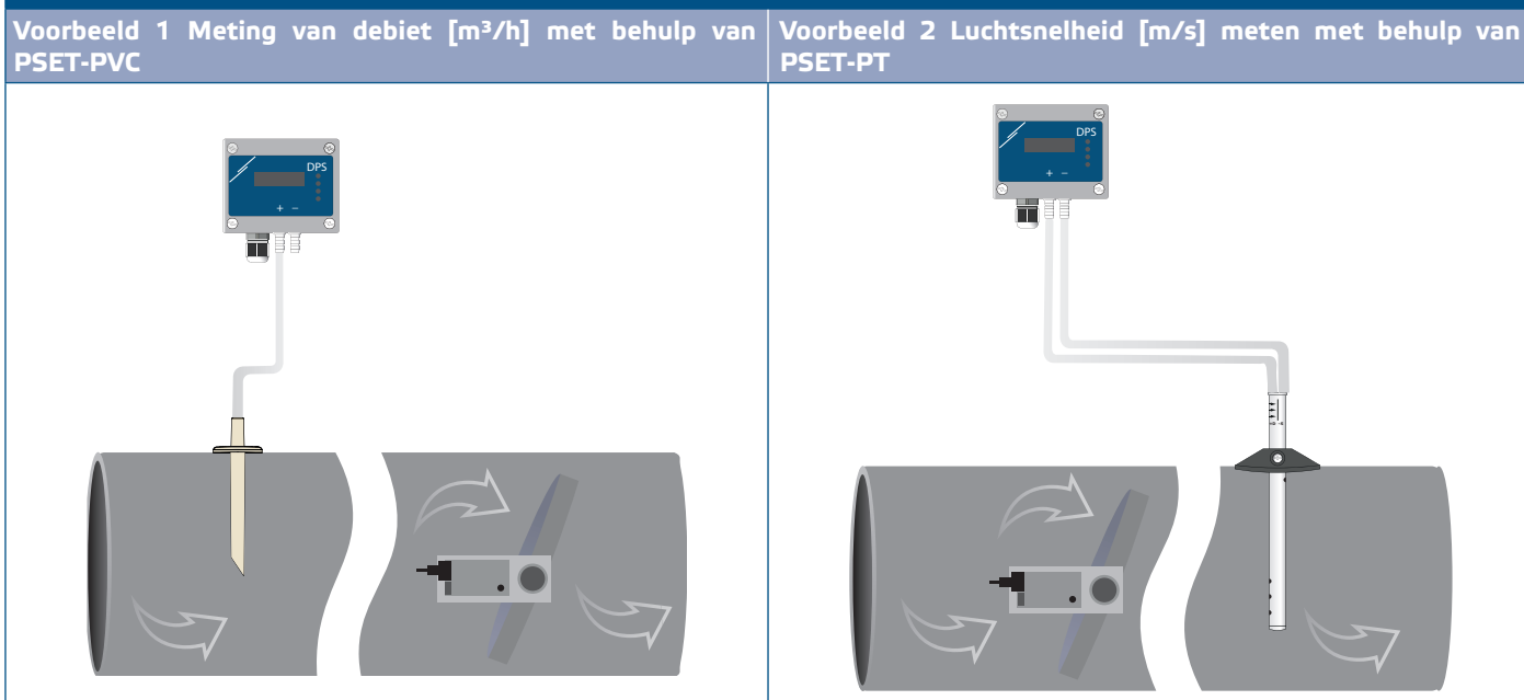
Fig. 4 Aansluiten met toebehoren
