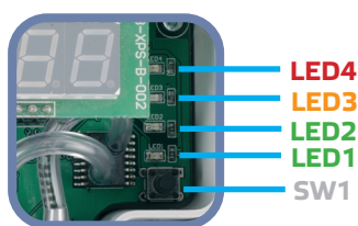
Fig. 7 Microschakelaar voor reset van de modbusregisters en voor de kalibratie van de sensor
