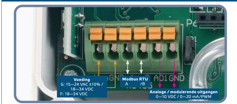
Fig. 3 Aansluitschema
