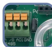
Fig. 5 Pull-up weerstand geactiveerd
