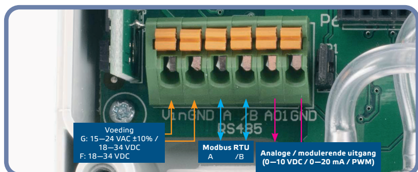
Fig. 3 Aansluitschema
