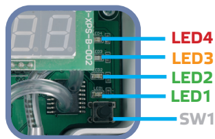
Fig. 8 Microschakelaar voor reset van de modbusregisters en voor de calibratie van de sensoren
