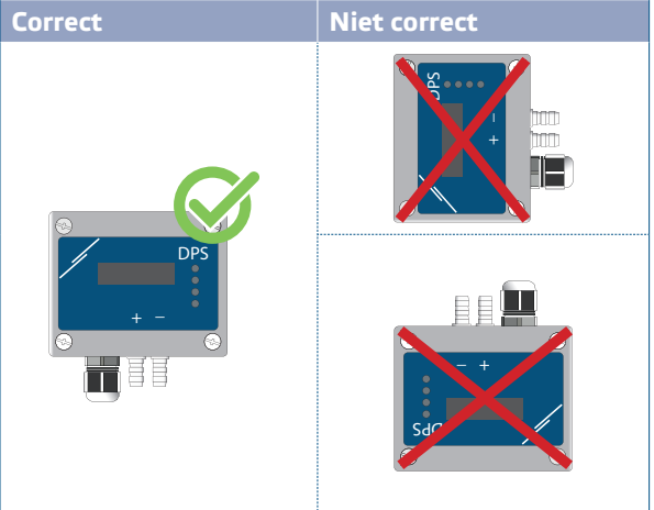
Fig. 2 Montagepositie
