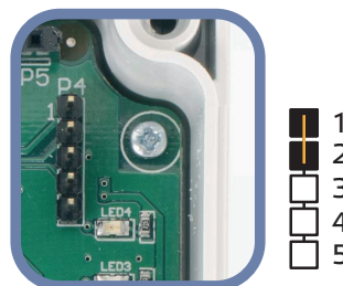
Fig. 10 Reset jumper voor Modbus communicatieregisters
