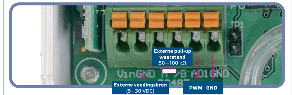
Fig. 6 PWM (Open collector) aansluiting (JP1 niet geplaatst)
