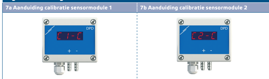
Fig. 7 Aanduiding calibratie
