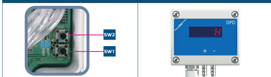
Fig. 8 Microschakelaar voor reset van de modbusregisters en voor de calibratie van de senso
