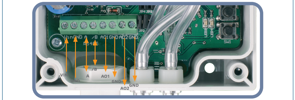
Fig. 3 Aansluitschema
