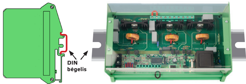
Fig. 2 Montavimo padėtis
