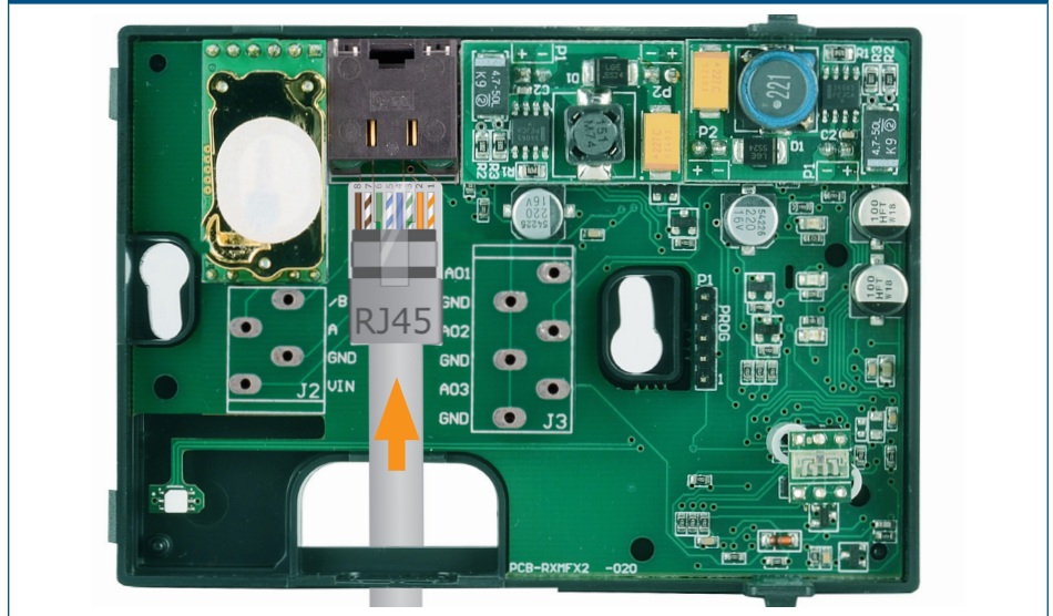
Fig. 4 Cablaggio
