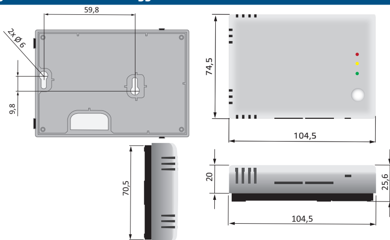
Fig. 2 Dimensioni di montaggio
