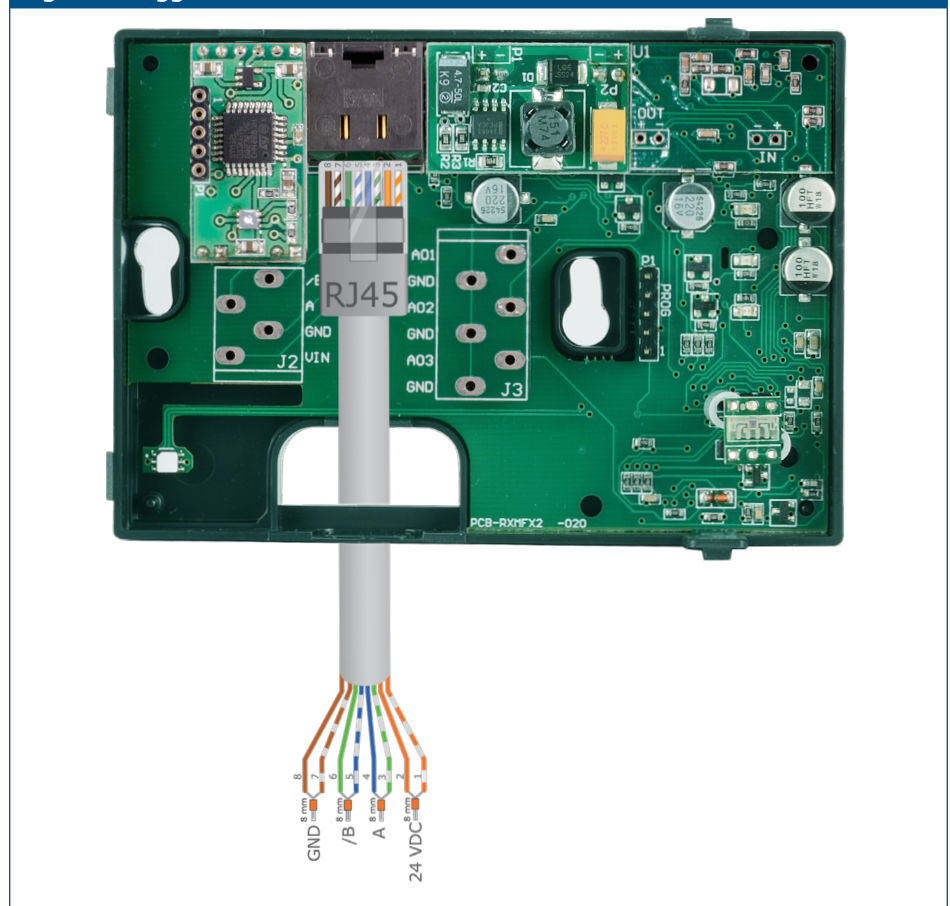
Fig. 4 Cablaggio
