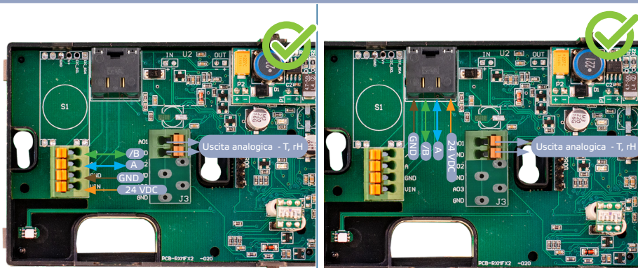
Fig. 4 Cablaggio e connessioni
