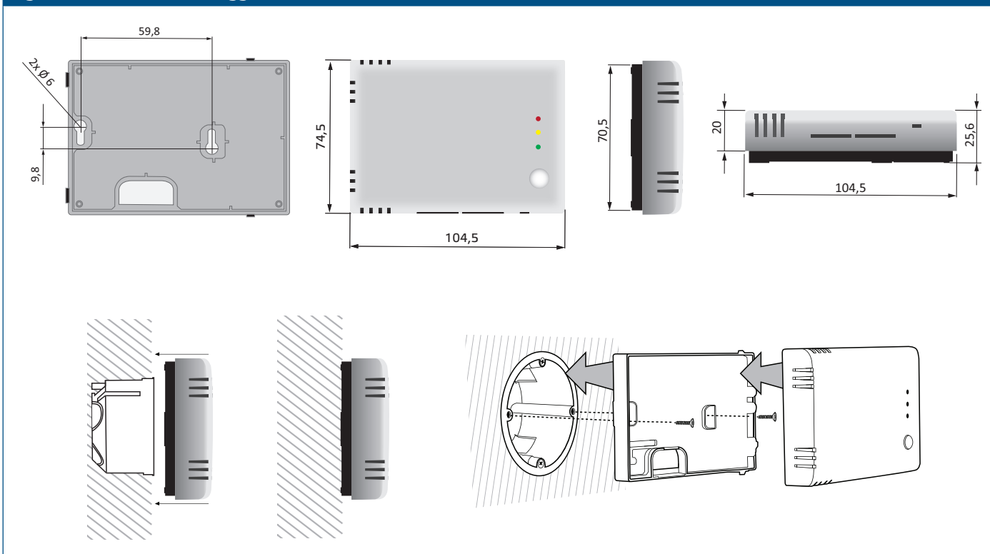
Fig. 2 Dimensioni di montaggio
