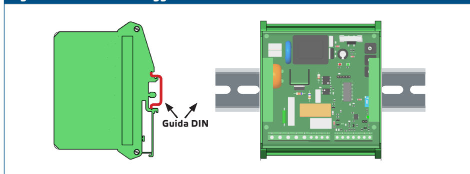
Fig. 2 Posizione di montaggio
