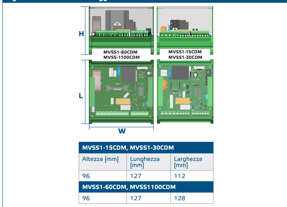
Fig. 1 Dimensioni di montaggio
