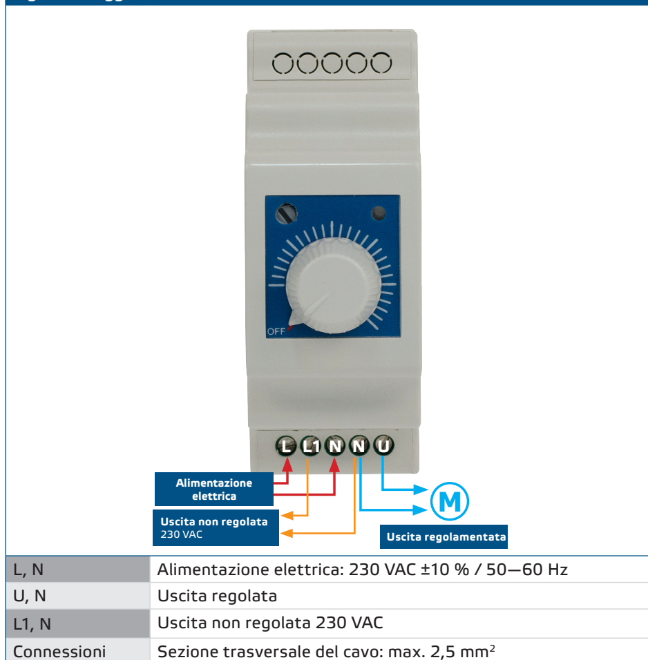
Fig. 1 Cablaggio
