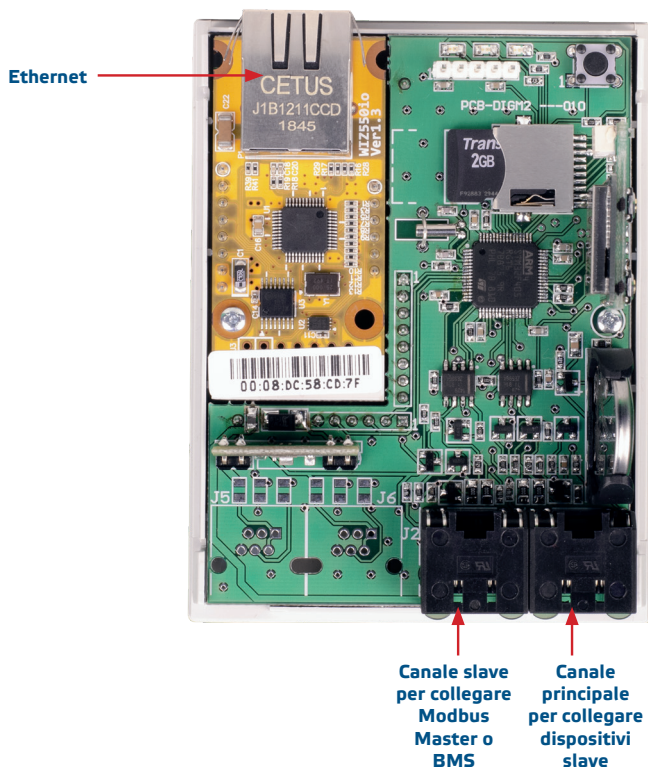
Fig.3 Cablaggio
