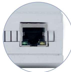
Vista dal basso - RJ45 PoM: Modbus RTU e alimentazione 24 VDC
