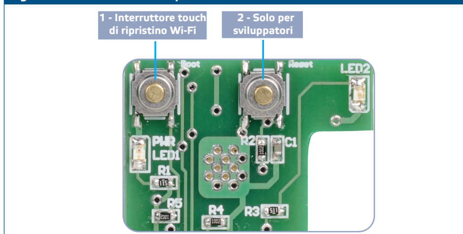
Fig. 5 Interruttore touch di ripristino Wi-Fi
