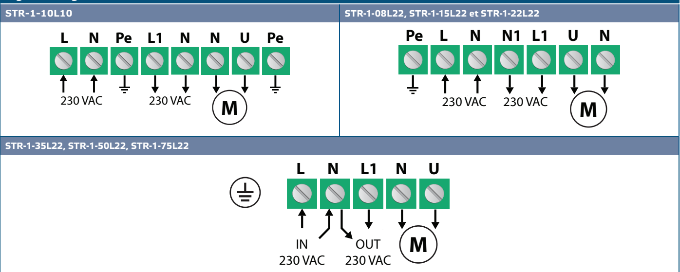
Fig. 3 Câblage et raccordements
