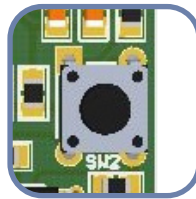
Fig. 10 Étalonnage du capteur et interrupteur tactile de réinitialisation du registre Modbus
