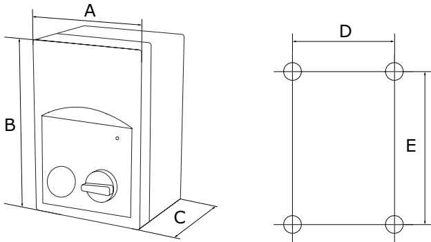
Fig. 1 Dimensions de montage
