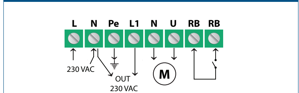
Fig. 3 Câblage et raccordements
