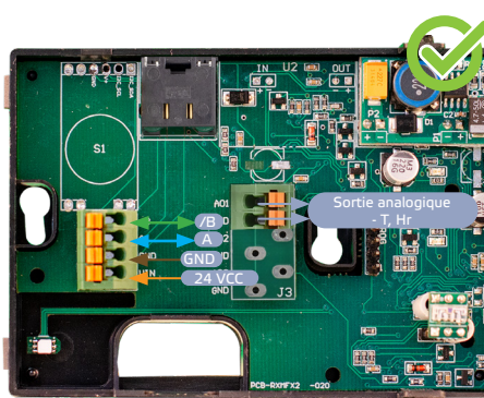
Fig. 4 Câblage et raccords
