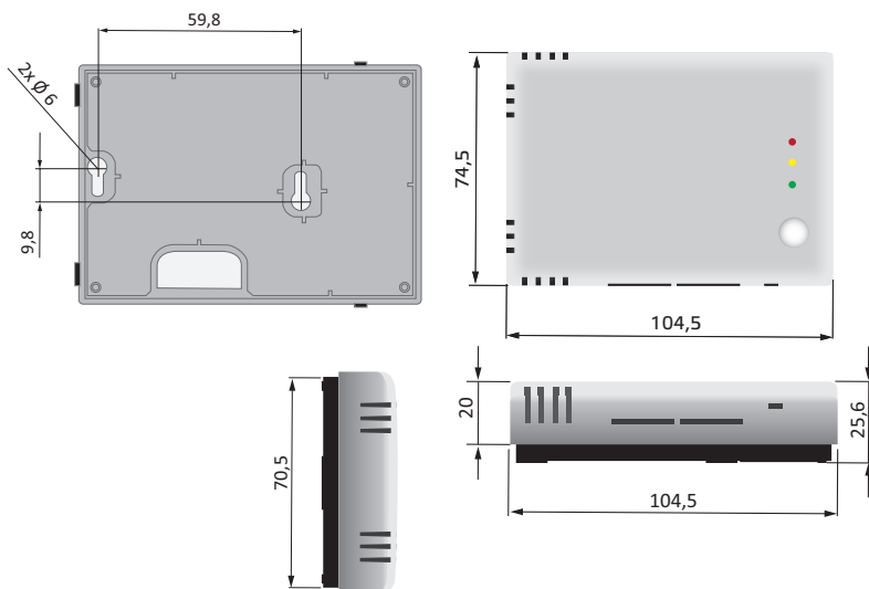
Fig. 2 Dimensions de montage
