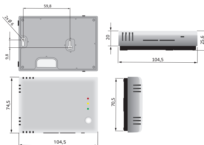
Fig. 2 Dimensions de montage
