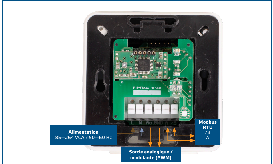
Fig. 1 Câblage et raccords
