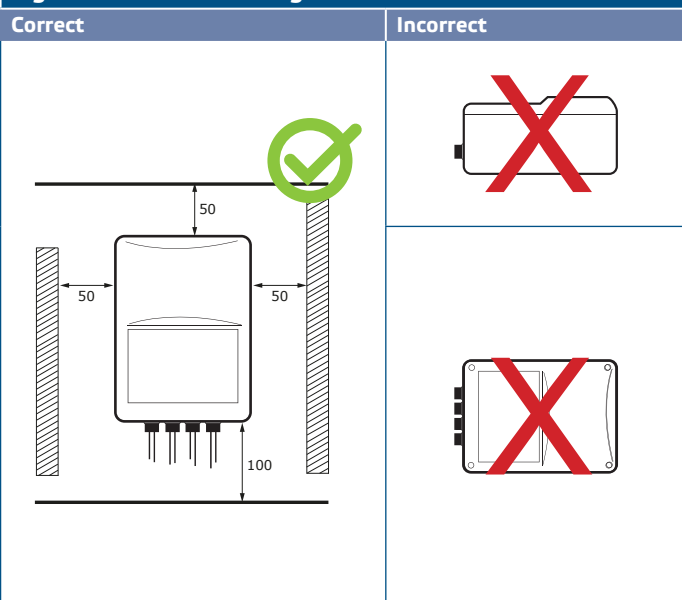
Fig. 2 Position de montage
