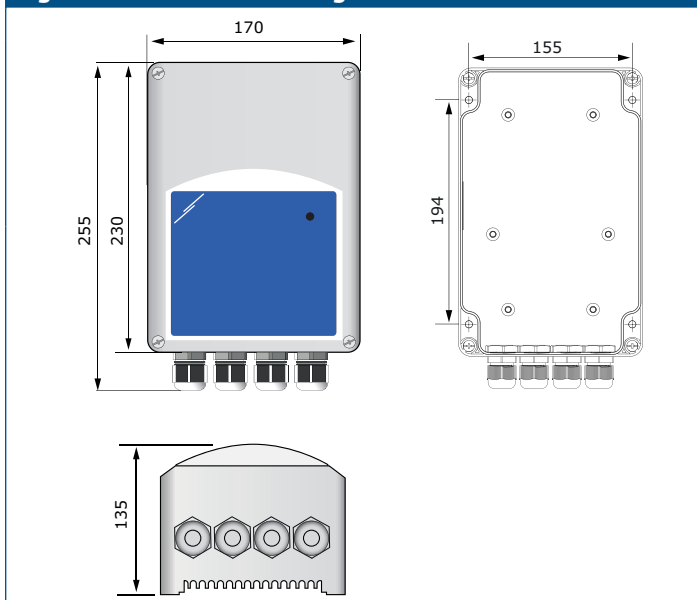
Fig. 1 Dimensions de montage
