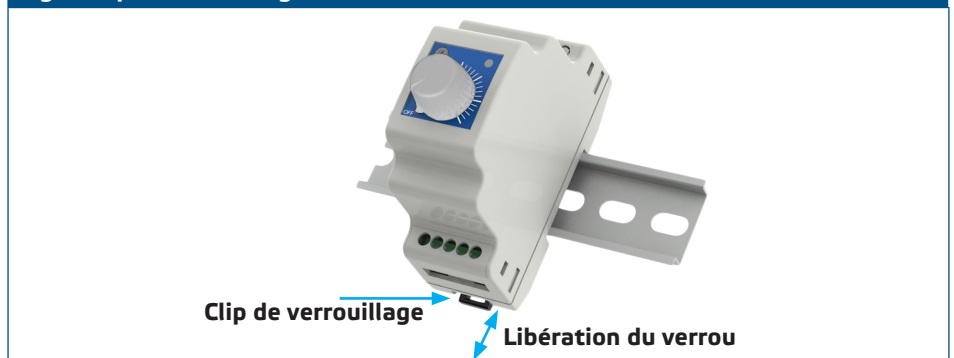
Fig. 2 Clip de verrouillage de rail DIN
