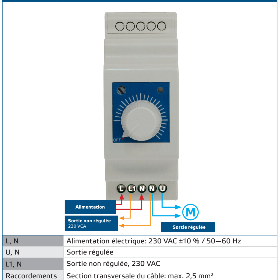
Fig. 1 Câblage
