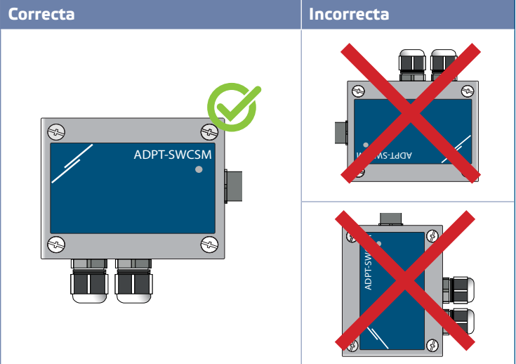
Fig. 4 Posición de montaje
