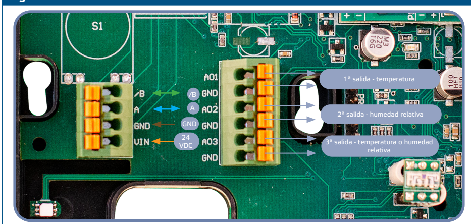
Fig. 4 Cableado
