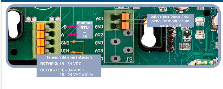
Fig. 4 Cableado
