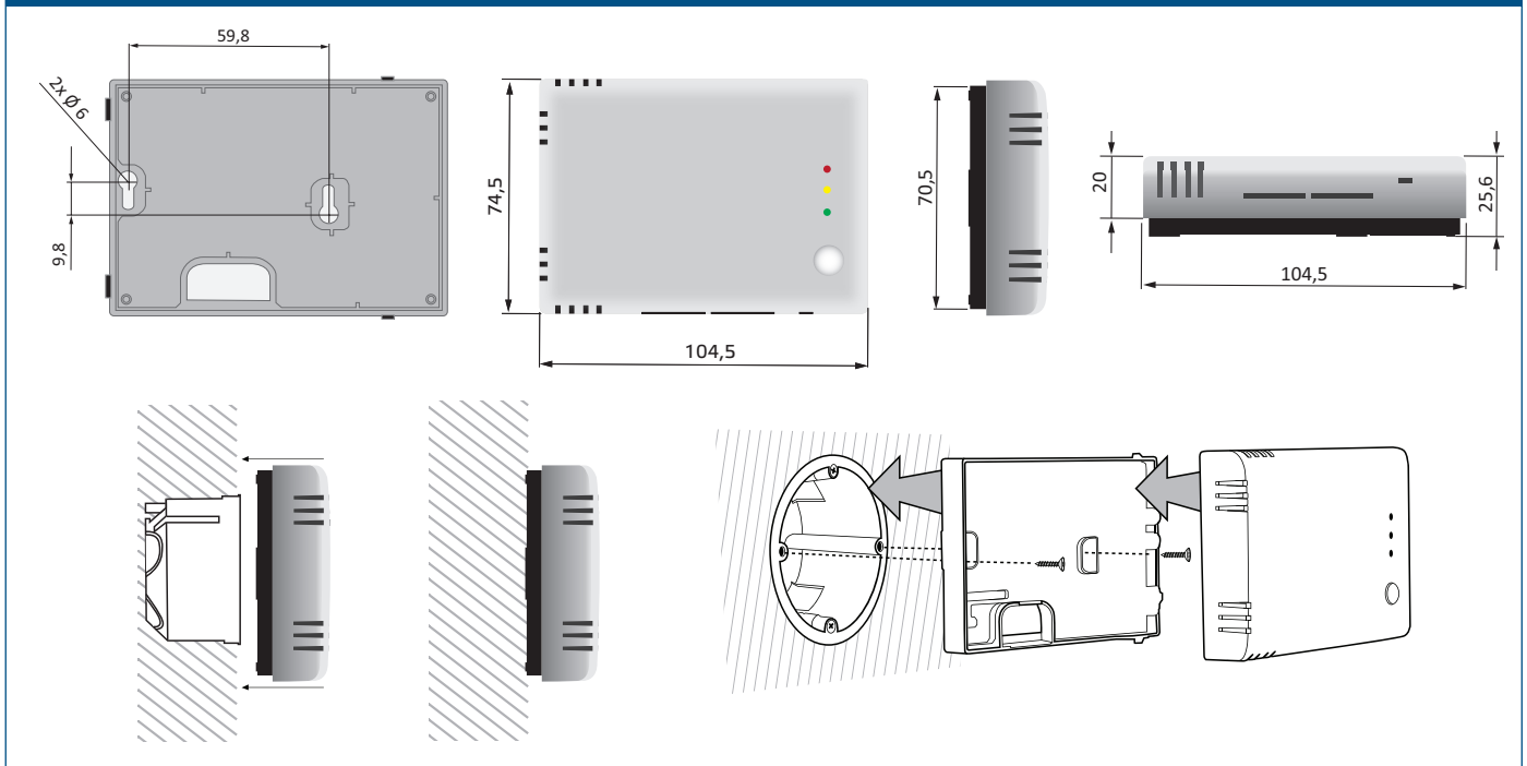
Fig. 2 Dimensiones de montaje
