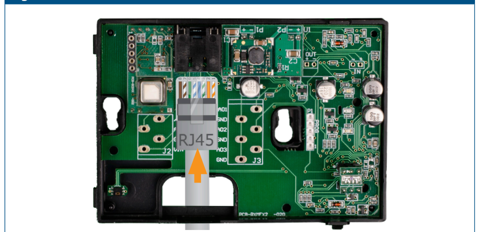
Fig. 4 Cableado
