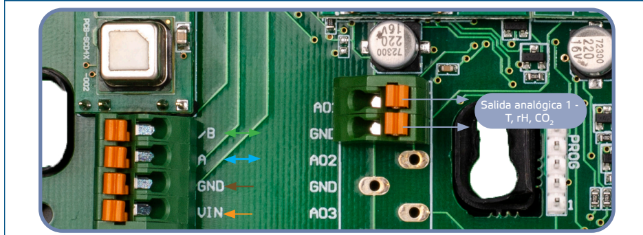
Fig. 4 Cableado
