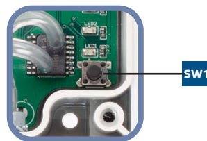
Fig. 6 Indicación de calibración y de reinicio del registro Modbus
