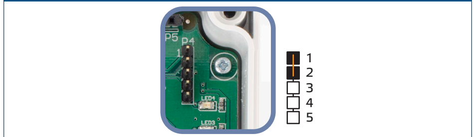
Fig. 8 'Jumper' de reinicio de los 'holding registers'
