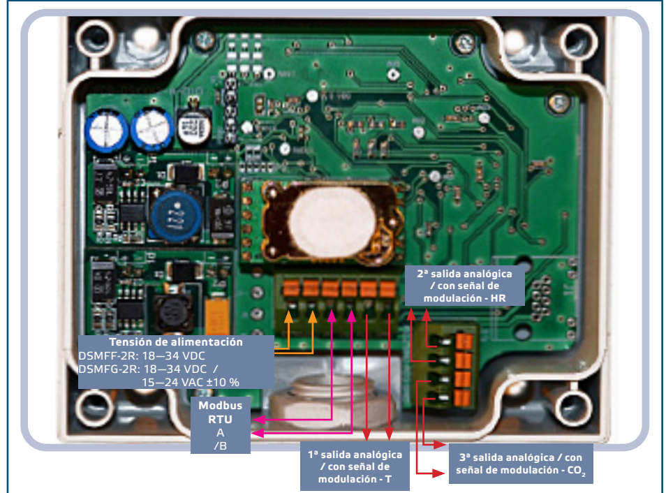
Fig. 4 Cableado y conexiones
