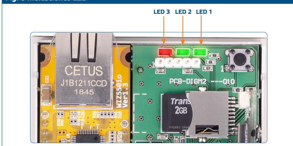
Fig. 6 Indicaciones LED
