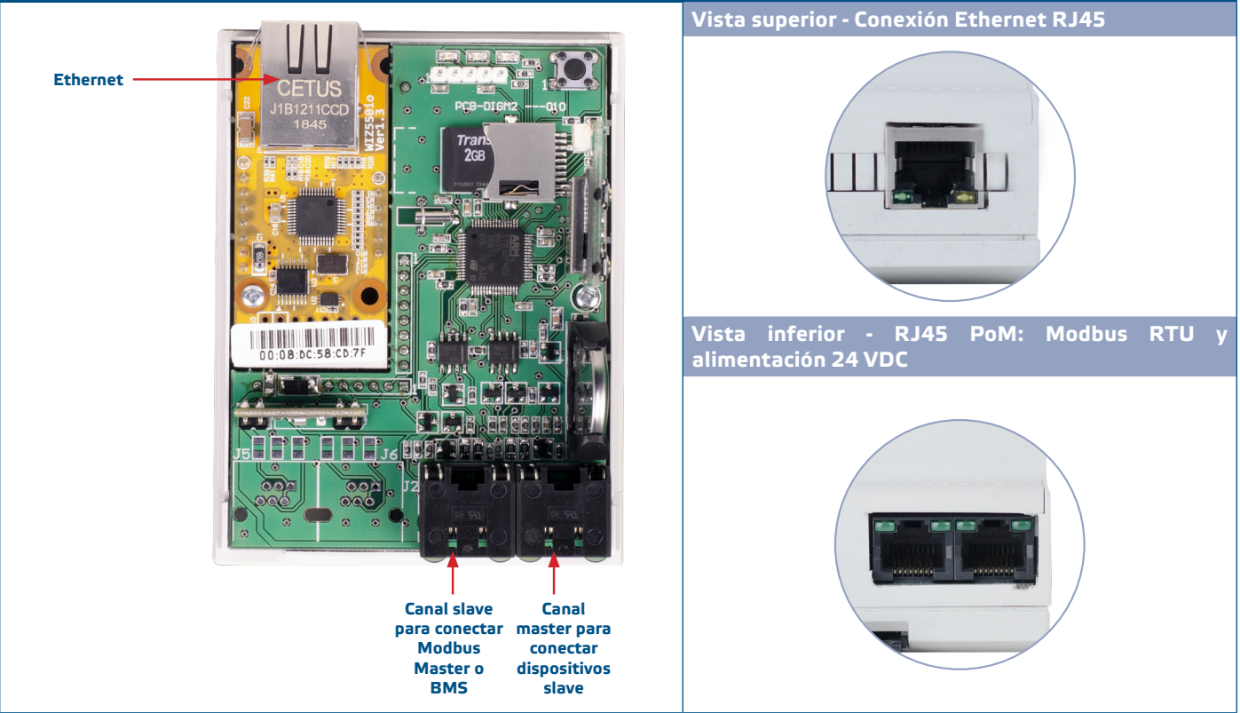
Fig. 3 Cableado
