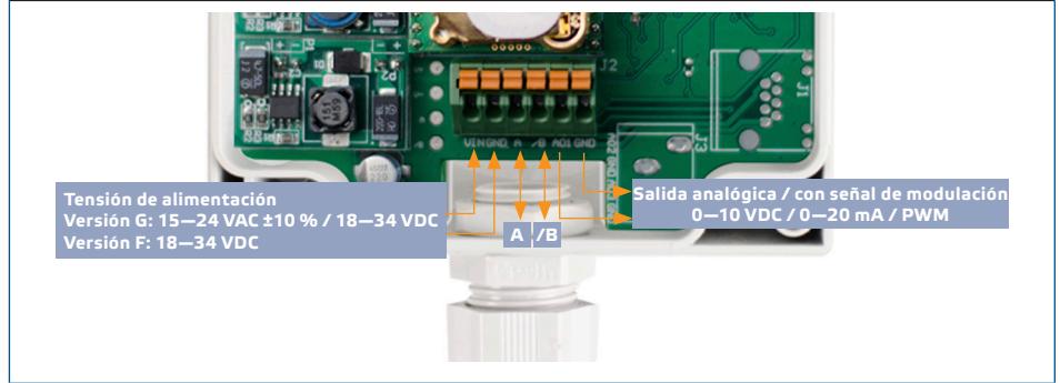
Fig. 4 Cableado y conexiones
