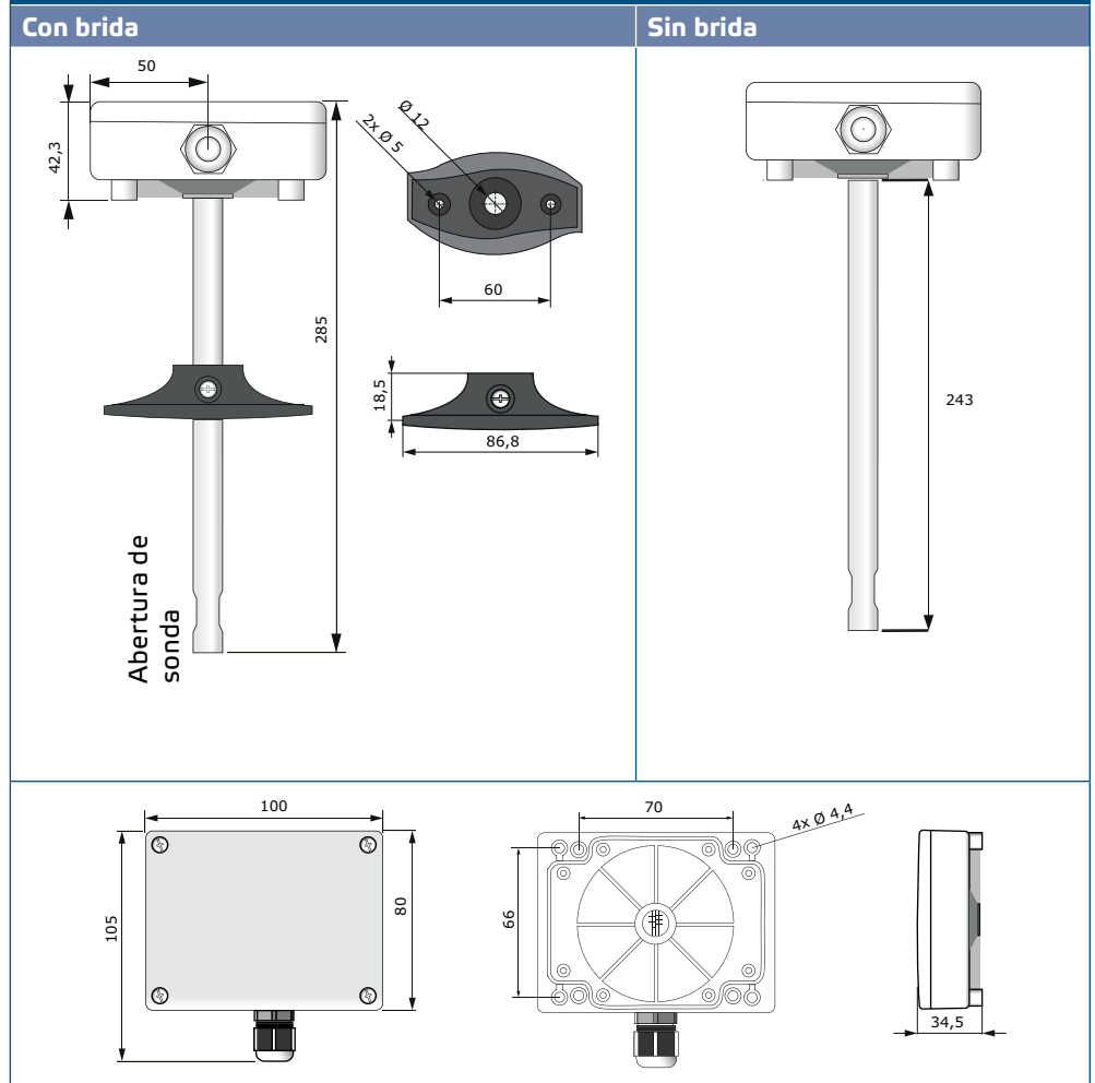
Fig. 1 Dimensiones de montaje
