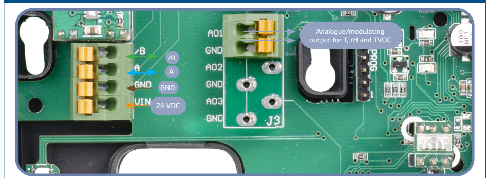
Fig. 4 Wiring
