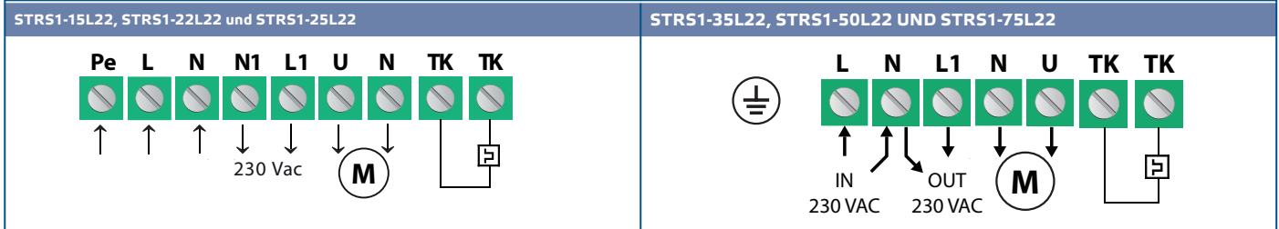
Fig. 3 Verkabelung und Anschlüsse
