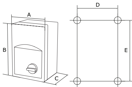
Fig. 1 Einbaumaße
