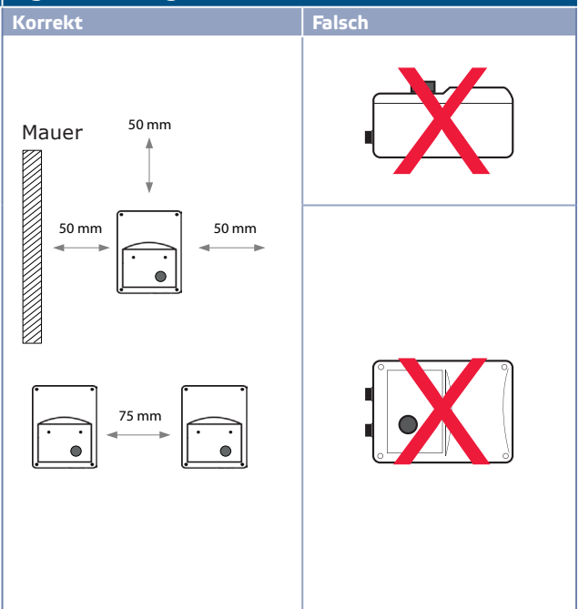
Fig. 2 Einbaulage
