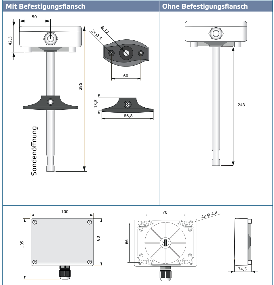
Fig. 1 Einbaumaße
