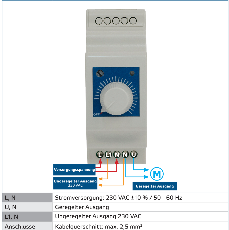
Fig. 1 Verdrahtung
