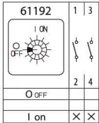
Schaltdiagramm 61192
