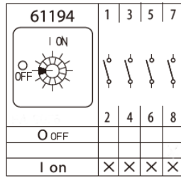
Schaltdiagramm 61194
