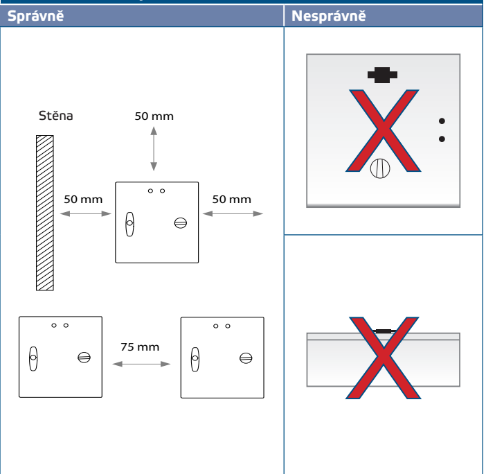
Obr. 2 Montážní poloha
