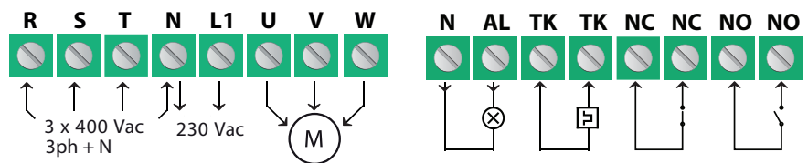
Obr. 3 Elektroinstalace a připojení
