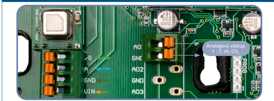
Obr. 4 Zapojení
