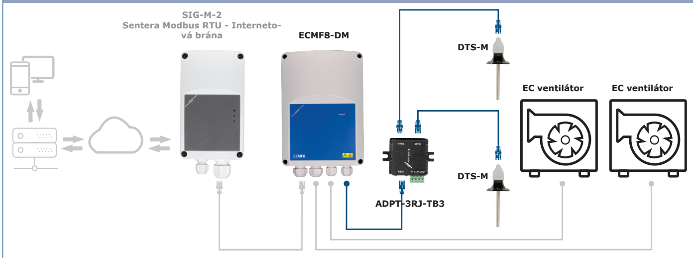
Příklad použití: ECMF8 + čidlo DTS, připojené k SenteraWebu pomocí brány Sentera
