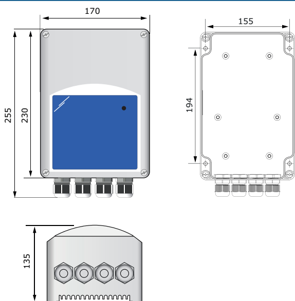
Obr. 1 Montážní rozměry
