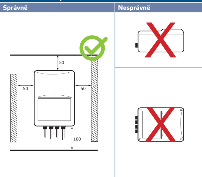
Obr. 2 Montážní poloha
