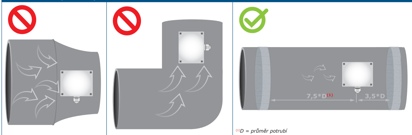
Obr. 3 Montážní požadavky
