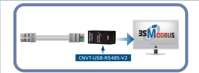
Фиг. 5 Свързване към 3SModbus с връзка RJ45
