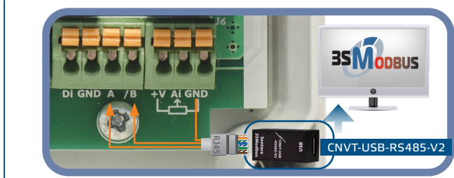
Фиг. 4. Свързване към 3SModbus с клеморед
