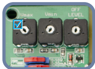
Фиг. 5 Тример за настройка на макс. обороти
