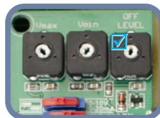
Фиг. 7 Тример на настройка на ниво на изключване
