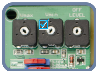
Фиг. 6 Тример за настройка на мин. обороти
