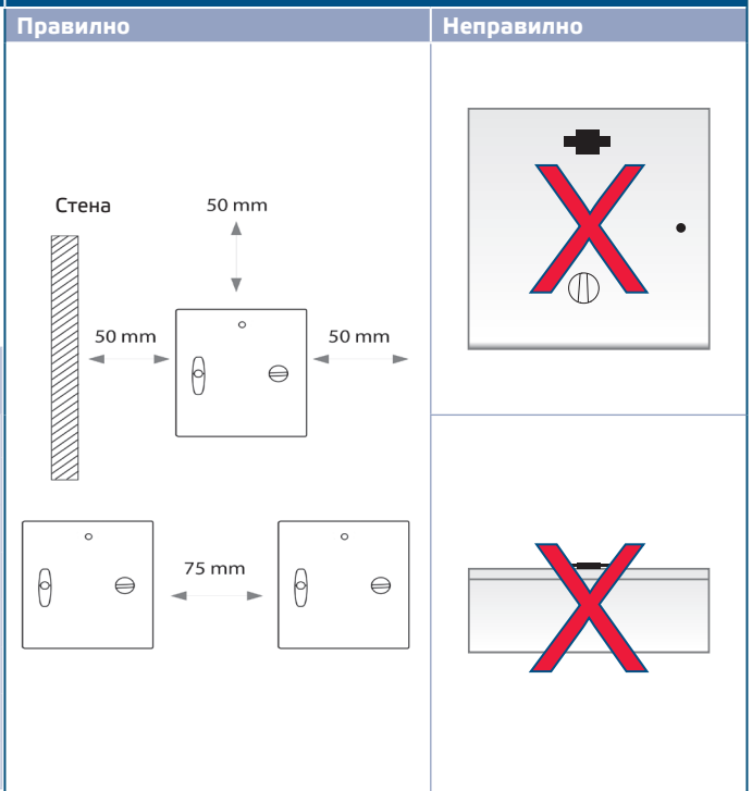
Фиг. 2 Положение за монтаж
