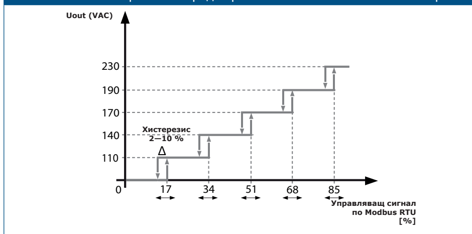
Фиг. 4 Автоматичен режим напред Управление от ниски към високи обороти
